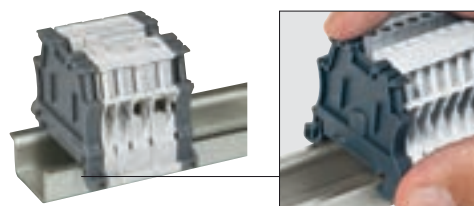
Торцевой стопор 0 375 10, безвинтовое крепление
