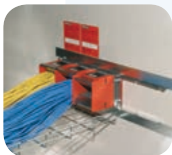
► ПРОХОД КАБЕЛЬНОЙ ТРАССЫ ЧЕРЕЗ СТЕНУ ПРИ ПОМОЩИ УНИКАЛЬНЫХ ОГНЕСТОЙКИХ МОДУЛЕЙ EZ-PATH
