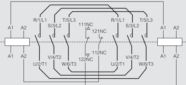
Типовая схема реверсивного контактора на основе CTX³ 9-150 А
